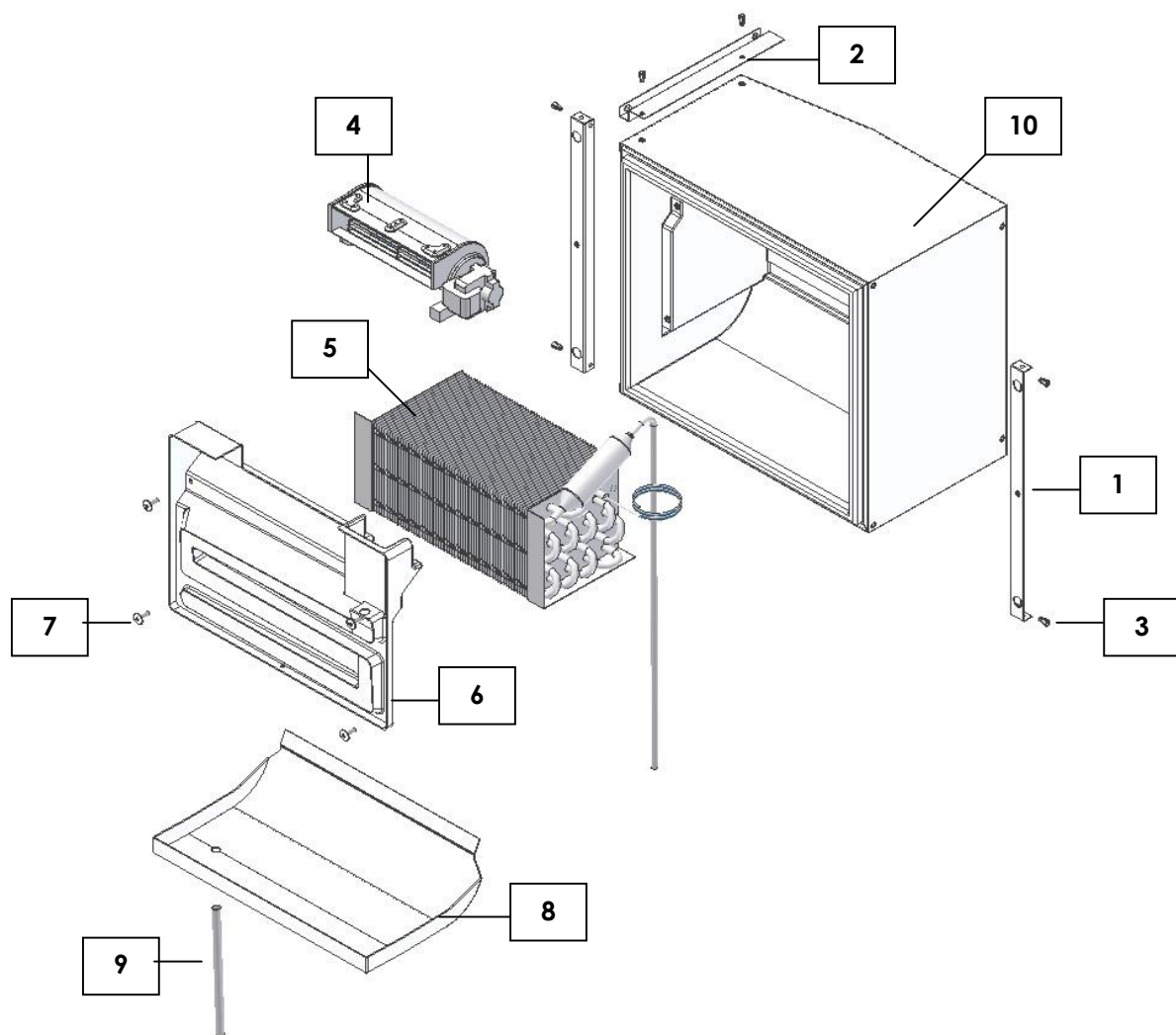
EVAPORATOR GROUP/GROUPE EVAPORATEUR/VERDAMPFEREINHEIT
