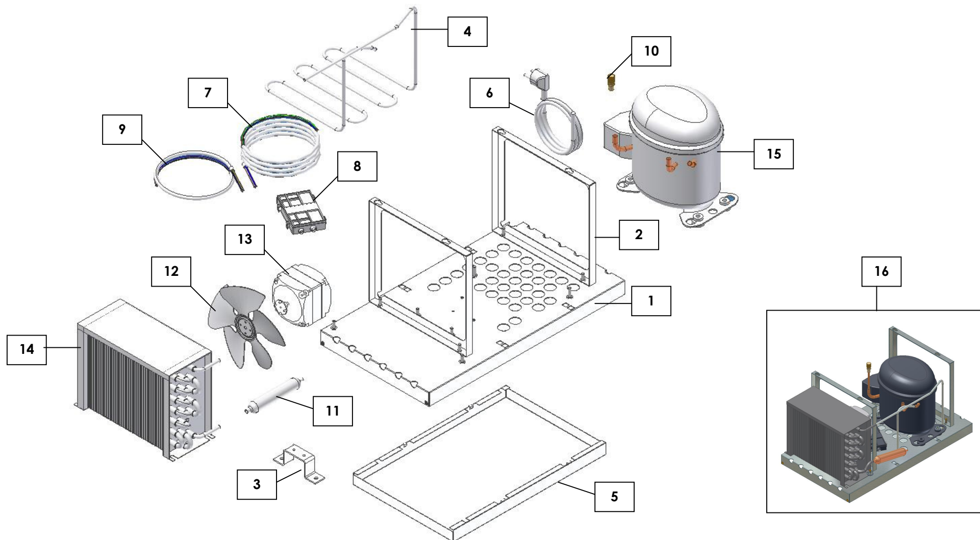
COMPRESSOR GROUP/GROUPE COMPRESSEUR/KOMPRESSOREINHEIT
