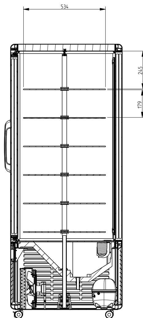
SEZIONE B-B
