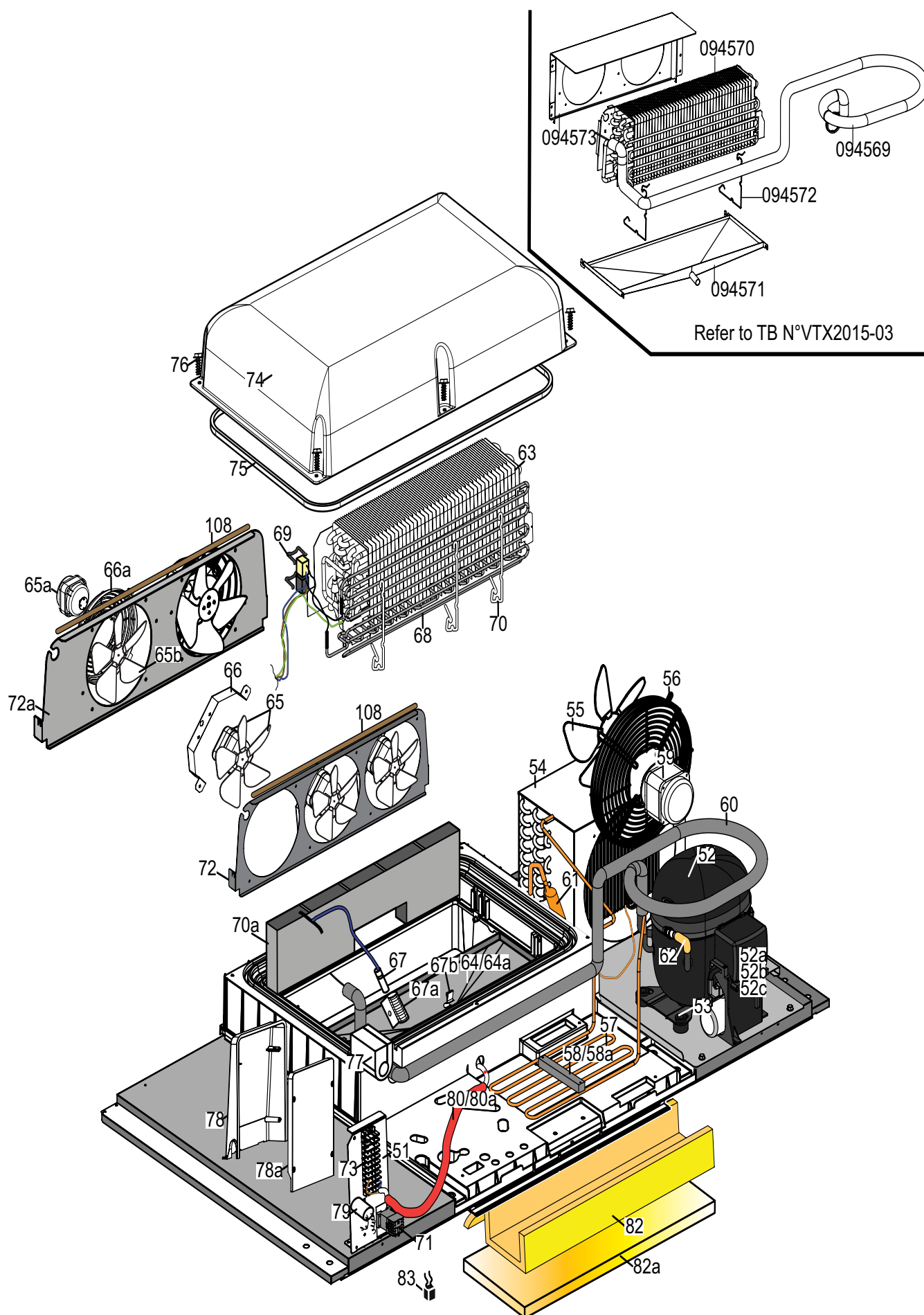
560112 gruppo freezer
